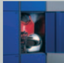
Bestell-Nr. 8370-203 Schließfachschrank mit 6 Fächern , Abt. Breite 400 mm (passend für Motorradhelme), extra tief, Maße (H x B x T in mm): 1950 x 820 x 590
